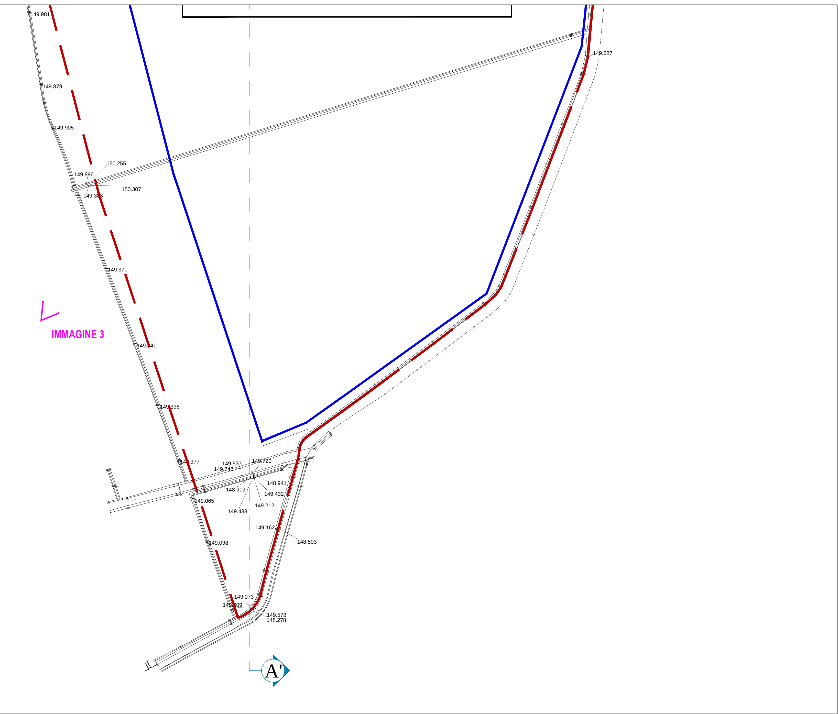
RILIEVO E PIANO QUOTATO - AMBITO SUD -SCALA 1.1000
